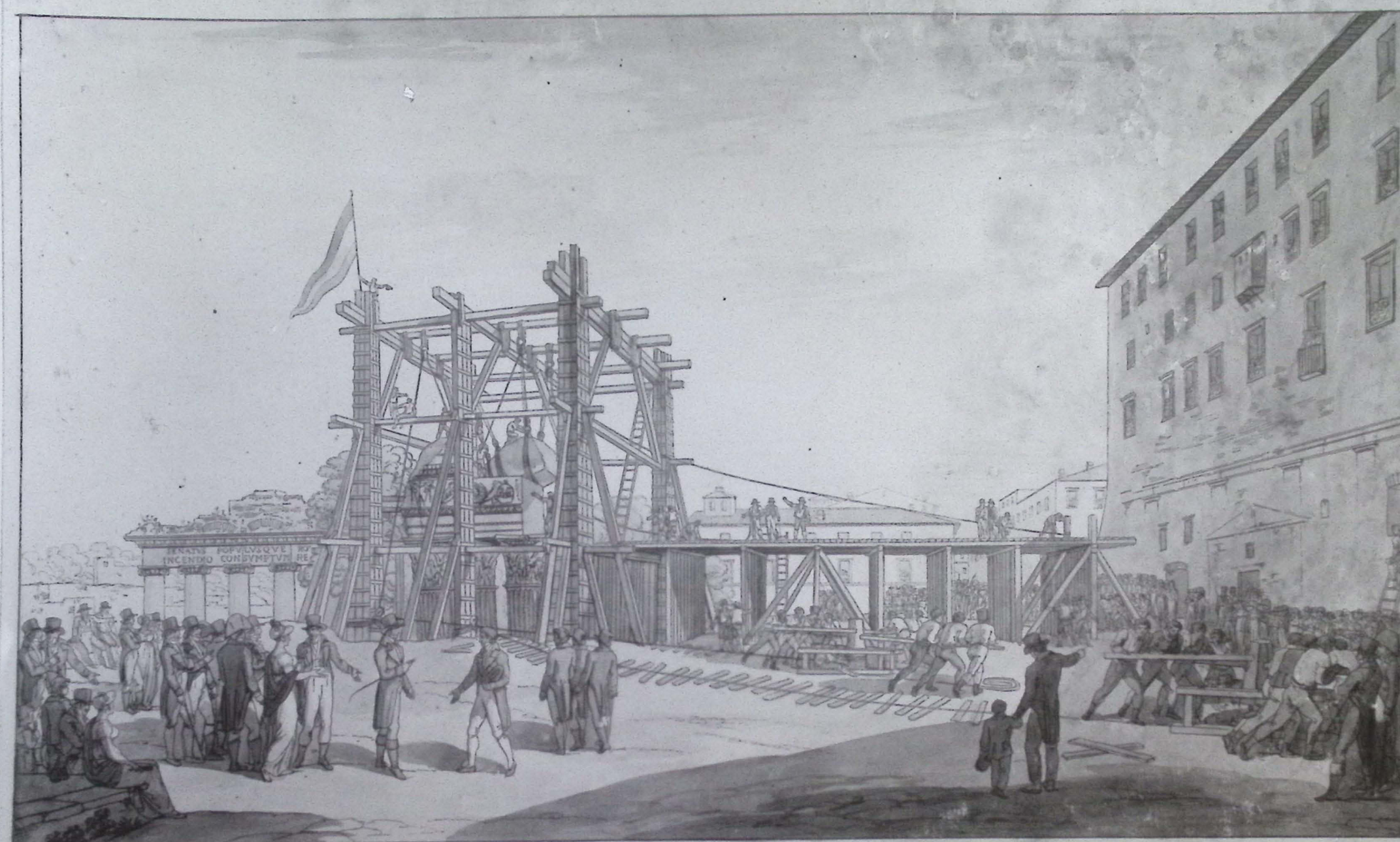
Disegno Prospettico del Castello per levare e opere le grandi Massi che formano l'Architrave, Fregio, e Cornice del Tempio di Giove Tonante e riaprobare le tre Colonne fuori di equilibrio, eseguite nel preciso momento dell'operazione del primo blocco
